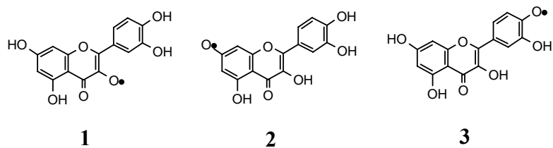
Figure 4 : Espèces susceptibles de réagir avec le dioxygène, activées en position 3-OH (forme n°1), 7-OH (2) ou 4'-OH (3) par le site actif de la LOX-3.
