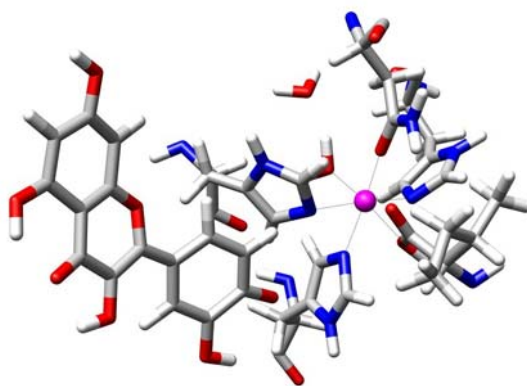
Figure 25 : Site actif de la LOX-3 dans la simulation ES3. Les deux premières molécules d'eau dans le canal sont représentées
