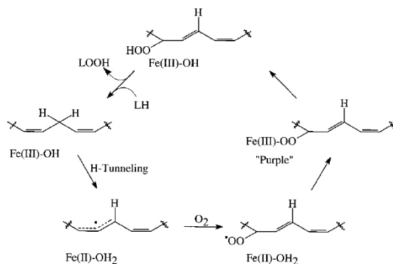
Figure 2 : Schéma de la dioxygénation des acides gras polyinsaturés au sein de la lipoxigénase 19 .
