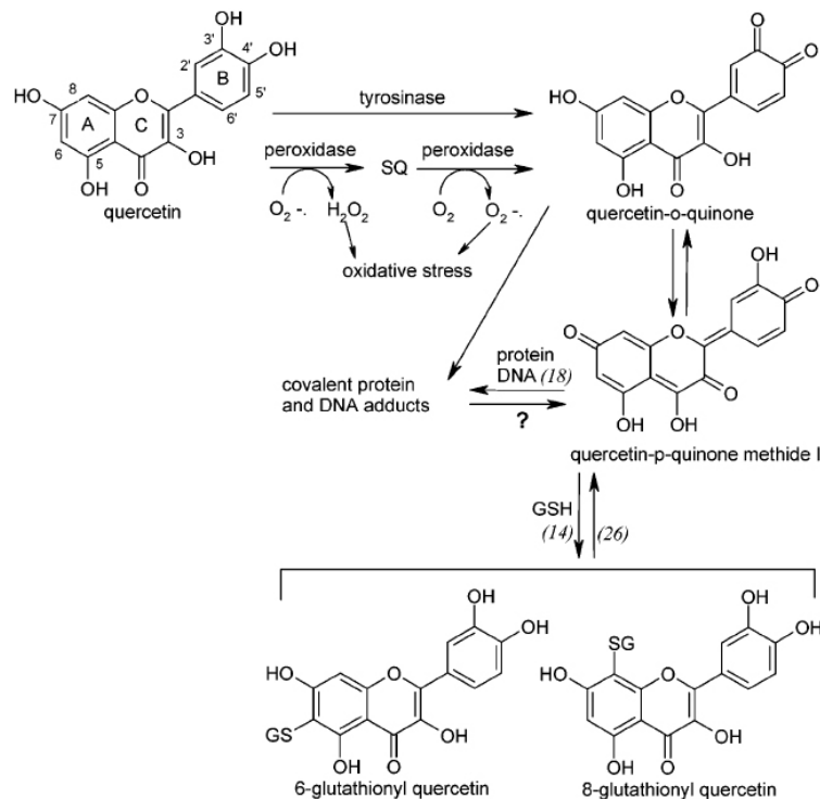
Figure 5 : relations proposées par Hester van der Woude et al. entre les formes actives de la quercétine et leur activité prooxydante 27 .
