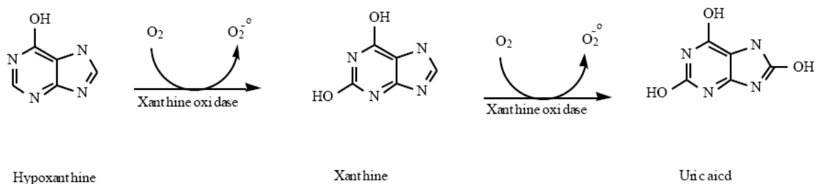
Figure 6 : processus enzymatique catalys  par la xanthine oxydase 21 .
