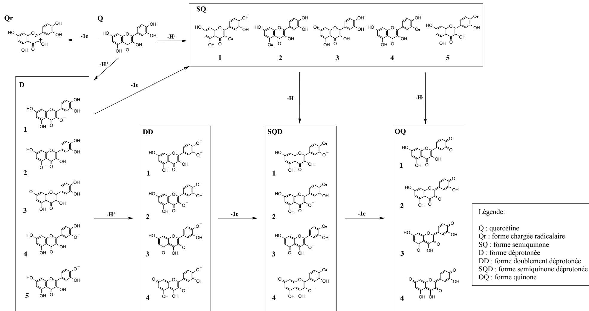
Figure 5 : Formes actives de la quercétine.
